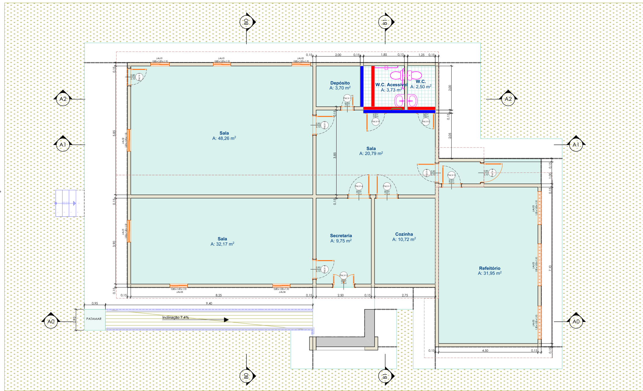
0. Pavimento Térreo Escala: 1:100
