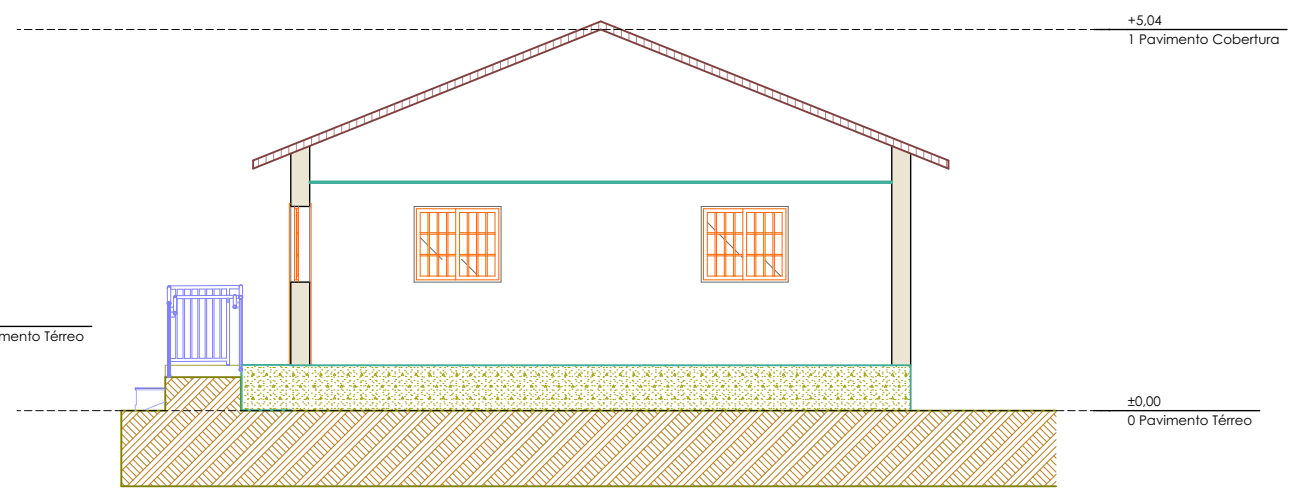
B1 Corte Escala: 1:100
