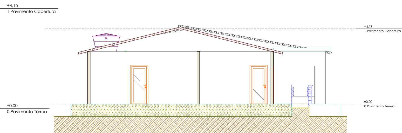
B0 Corte Escala: 1:100
