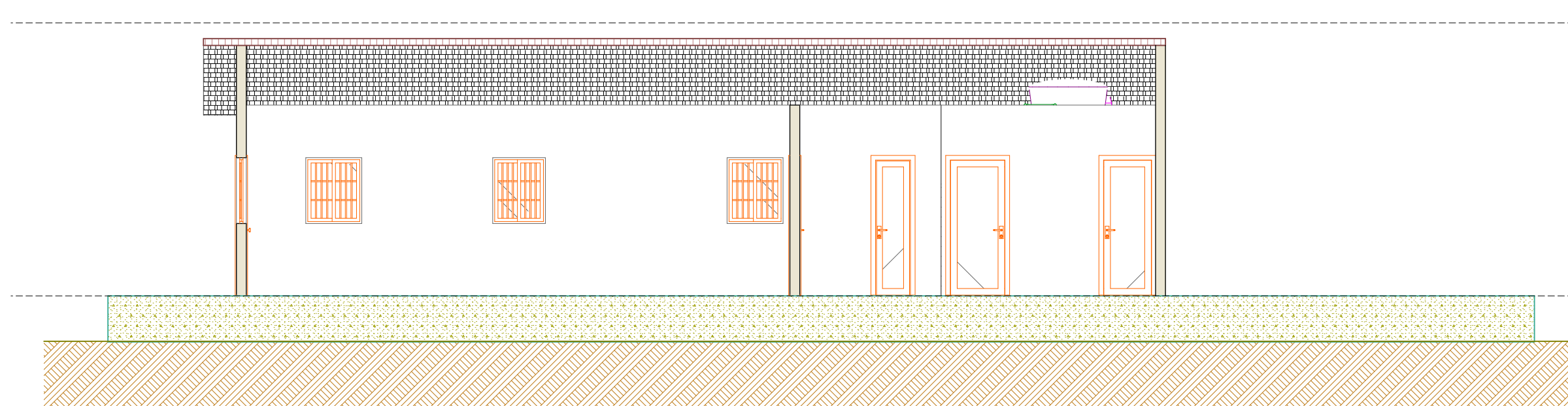
A1 Corte Escala: 1:75
