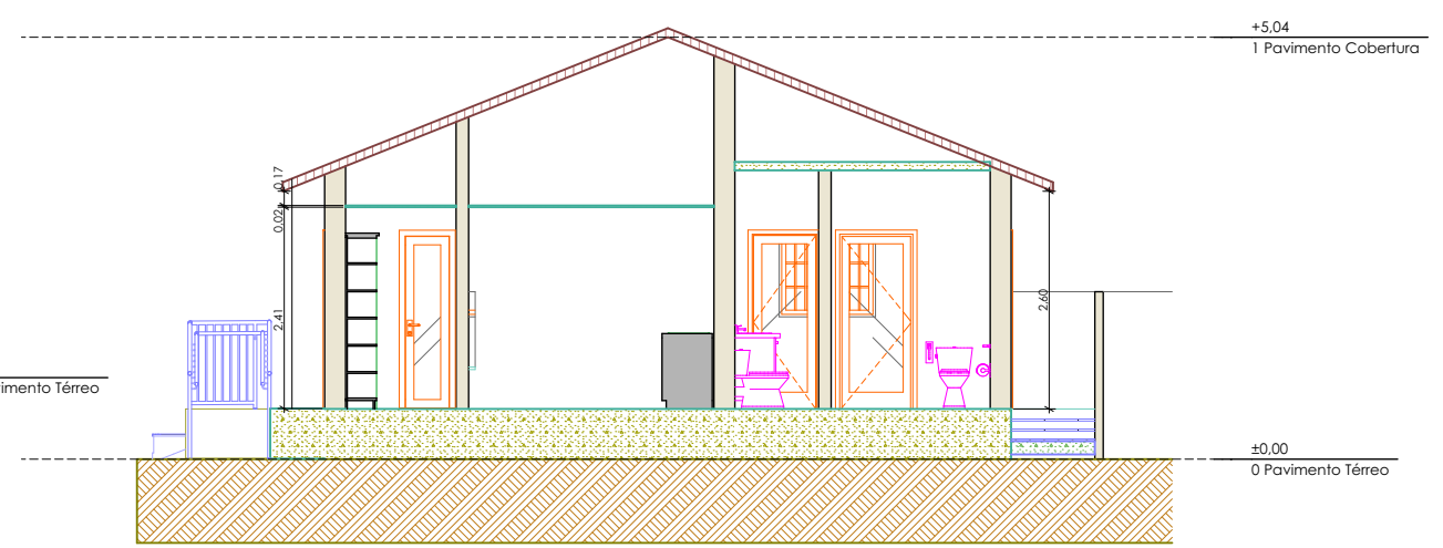
B0 Corte Escala: 1:100
